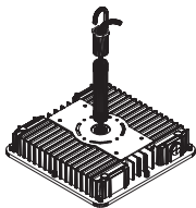
Hook 吊杆安装
